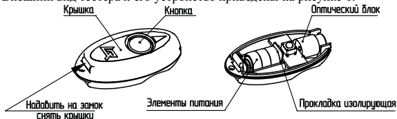
Рисунок 1 – Внешний вид тестера и его устройство
