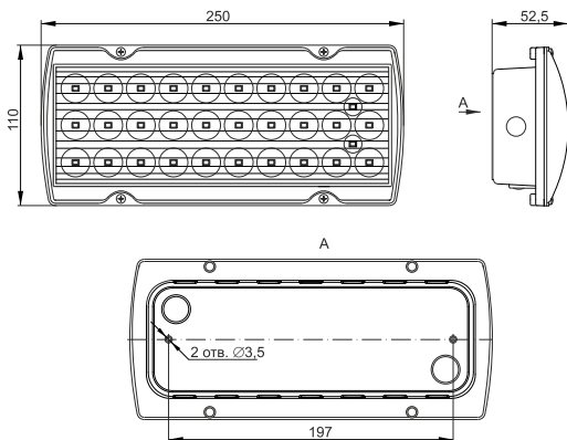
Рисунок 3 – ДПА 2105-С
