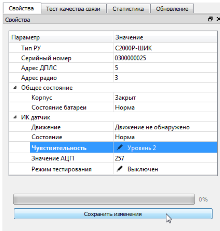
Рисунок 2.15 Настройка работы РУ
