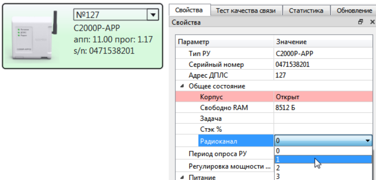
Рисунок 2.12 Выбор РЧ канала
