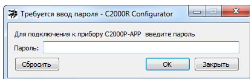
Рисунок 2.24 Запрос пароля
