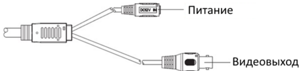
Рис. 1 Коммутационный кабель
