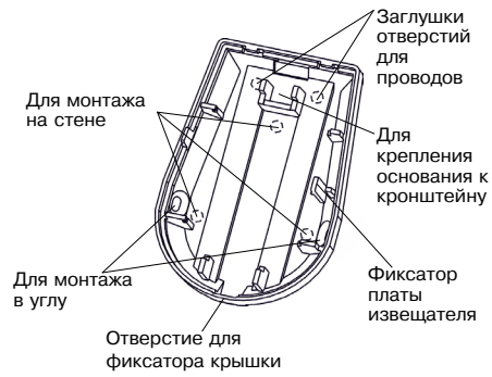
Рисунок 2 – Основание извещателя
