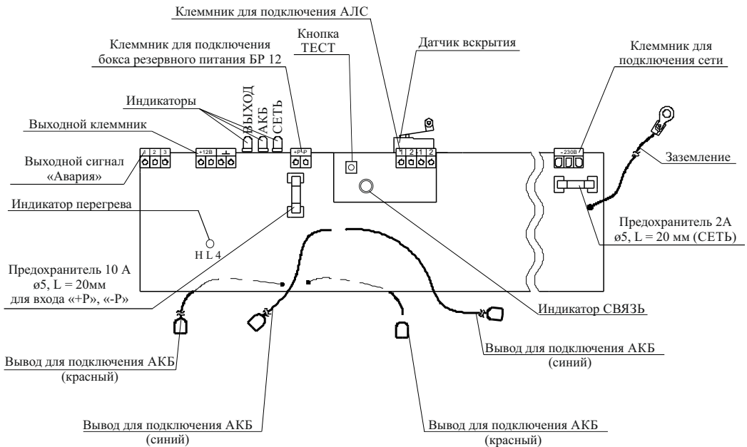
Рисунок 1 – Плата источника
