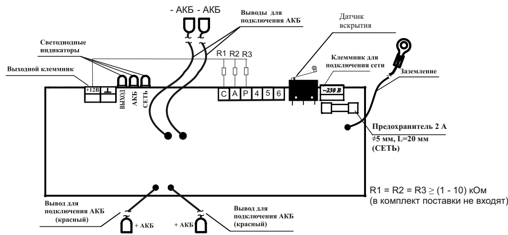
Рисунок 1 - Плата источника
