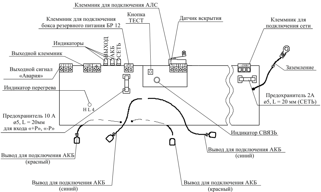
Рисунок 1 – Плата источника
