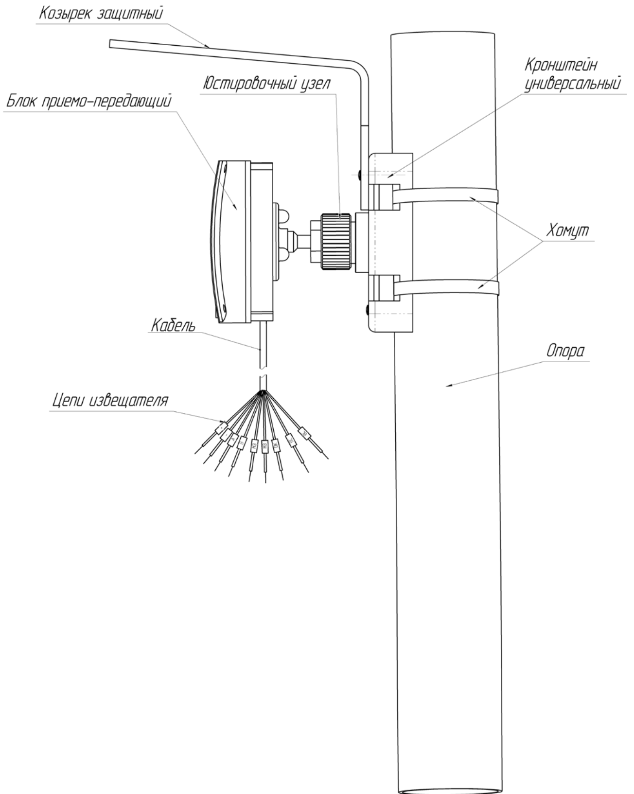
Рисунок 2.1 – Внешний вид блока приемо-передающего «АГАТ-6-24», установленного на опоре
