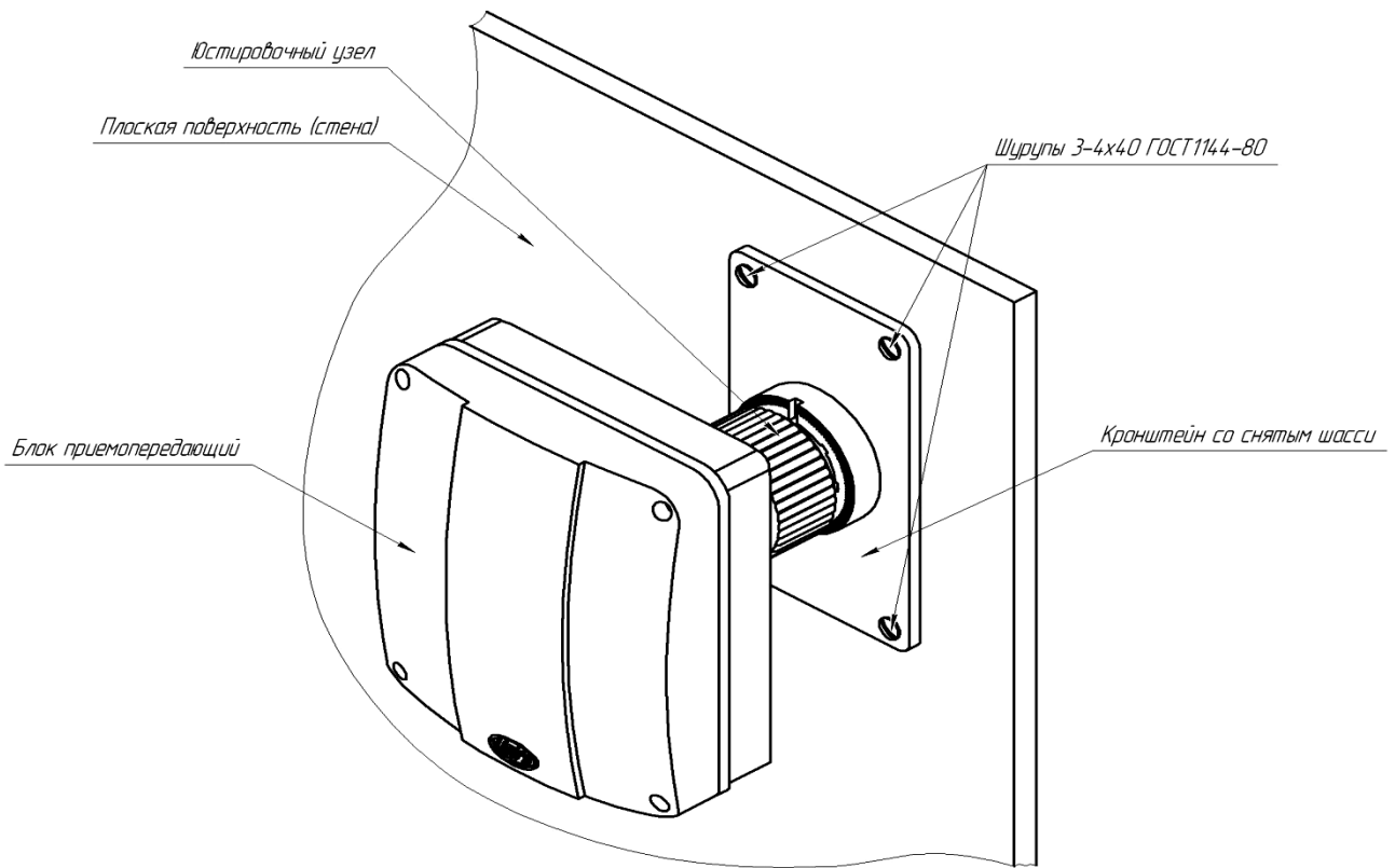
Рисунок 2.2 – Внешний вид блока приемо-передающего, установленного на плоской поверхности (стене)
