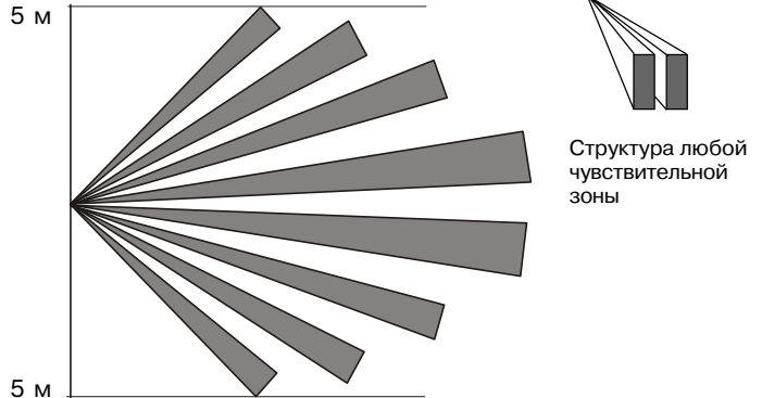
Рис. 1. Диаграмма зоны обнаружения
