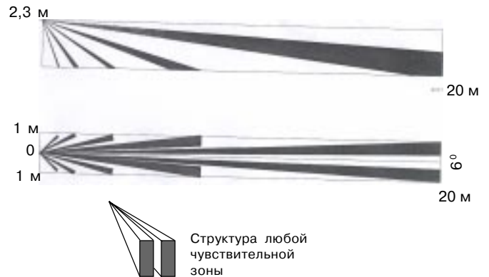
Рис. 1. Диаграмма зоны обнаружения
